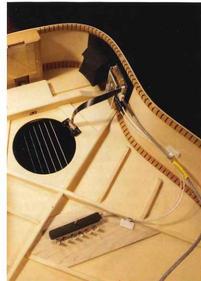
上記のギター内配線写真は、システム全体がわかりやすく見えるようにした配線イメージです。
